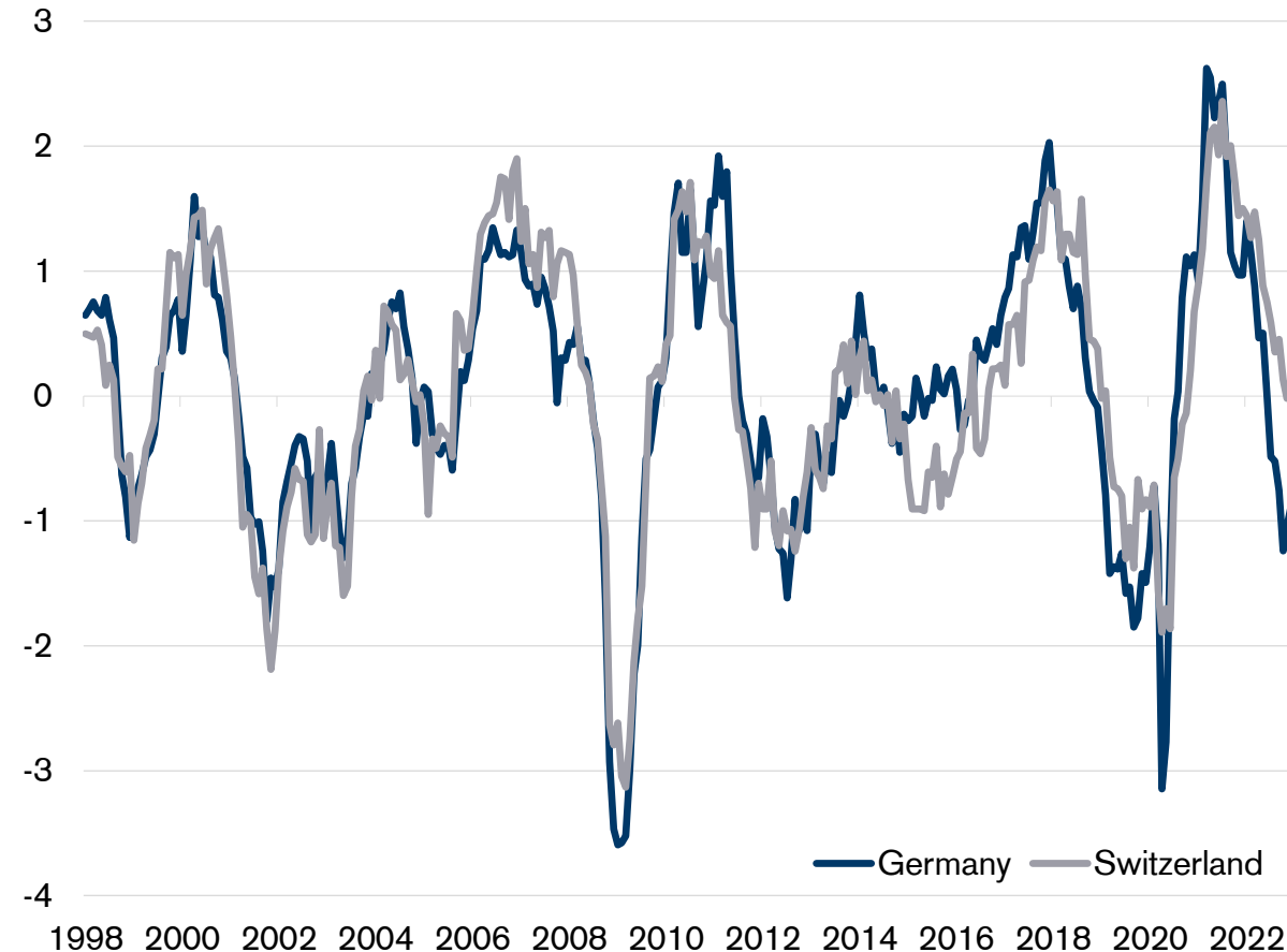
PMI, standardisiert
